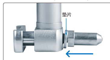
测头安装(245-050-11)
