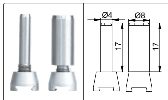
夹柱(标配)
