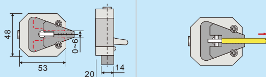
楔形夹头(货号: DF-WT1)
