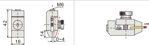
平夹头(货号: DF-FC2)
