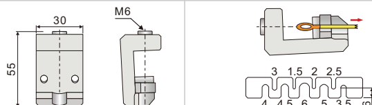
楔形夹头(货号: DF-WT1)
