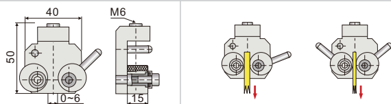
多用偏心夹具(货号: DF-CG2)
