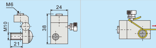
线缆端子夹头(货号: DF-TWG1)
