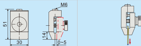
偏心夹头(货号: DF-CG1)
