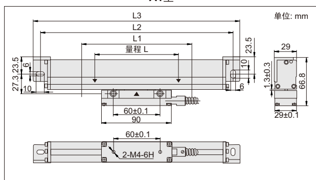
A1型
